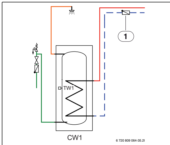
Мал. 9 Бак-водонагрівач
